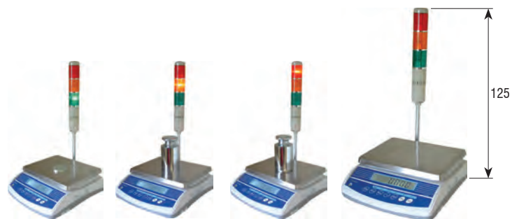
Verde < limit Amarelo = limit Vermelho > limit Semáforo com a função limites e sinal acústico
