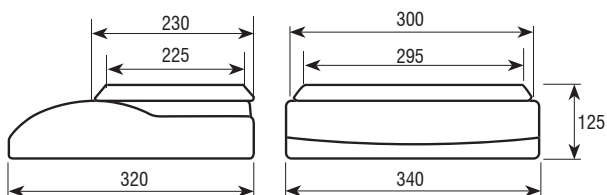
Dimensões (mm)
