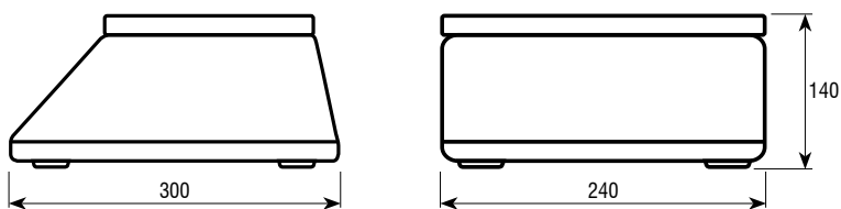
Dimensiones (mm)
